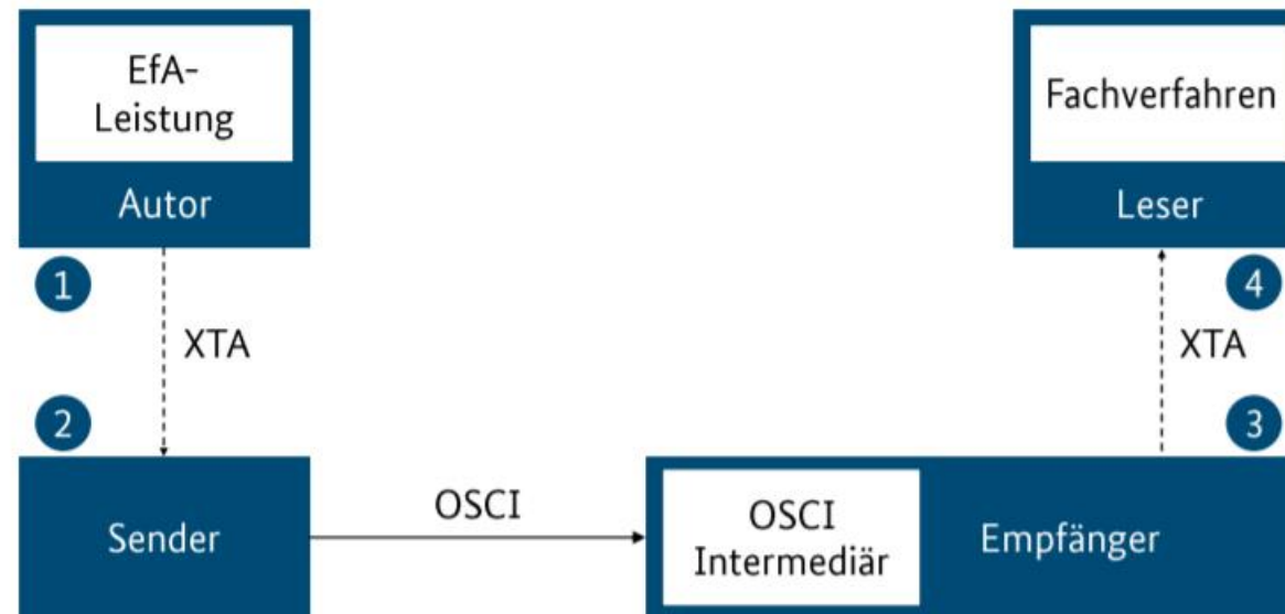
Abbildung 7: Schematische Transportinfrastruktur nach dem 4-Corner Model
